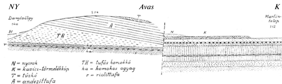
2. ábra. Ideális szelvény az Avason át a Danyivölgy és a Martintelep közt...
