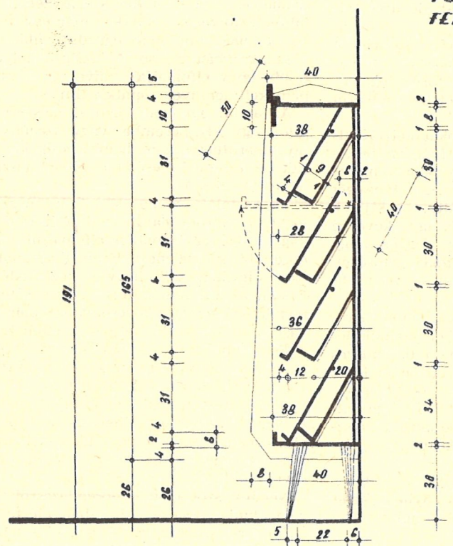
METSZET M = 1:20
