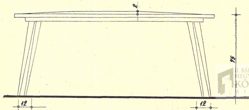
ELÖLNÉZET M= 1-20
