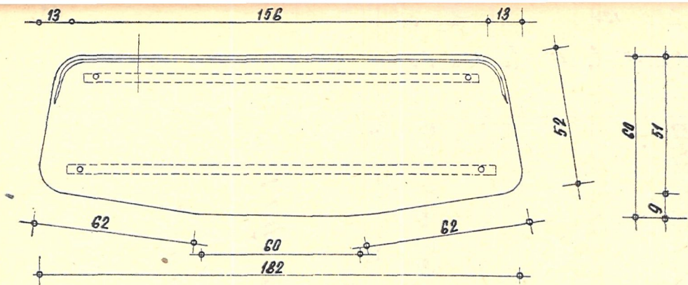
FELÜLNÉZET M- 1-20
