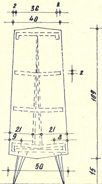
OLDALNÉZET M-1:20
