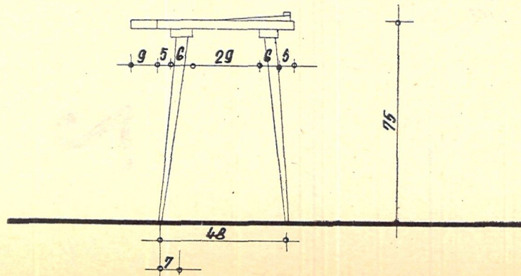
OLDALNÉZET M- 1-20
