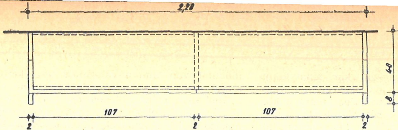
FELÜLNÉZET M = 1:20
