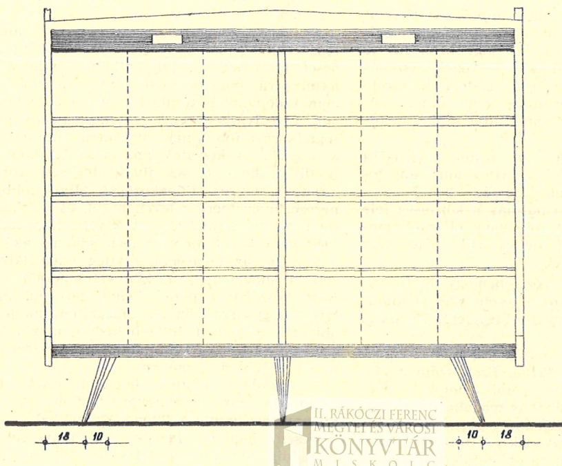
ELÖLNÉZET M = 1:20
